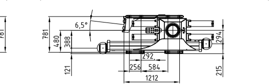
Seifensitz 02 universal rechts & links Side seat 02 universal right & left
